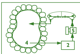
1. Pompa con filtro a reticella 2. Filtro 3. Pompa 4. Alimentazione a caduta 5. Filtro pressurizzato
